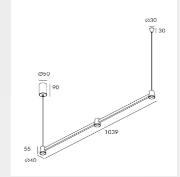
CONI Pendant Lamp
