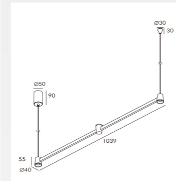
CONI Pendant Lamp
