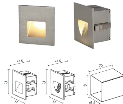
WL7572R & WL75723X0.7W
